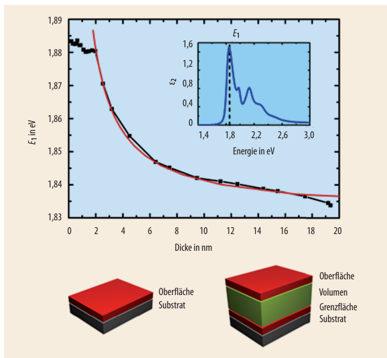
Abb. 6 Die Energie des ersten Peaks im Absorptionsspektrum von Pentacene (Inset, [13]) skaliert näherungsweise reziprok mit der Filmdicke D . Ursachen sind das geänderte Verhältnis von Grenzfläche zu Volumen (Schemazeichnung) sowie Unterschiede in der lokalen Umgebung eines Moleküls [10].
