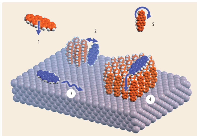
Abb. 1 Beim Wachstum einer atomaren oder molekularen Schicht spielen verschiedene Elementarprozesse eine Rolle: Absorption/Desorption (1), Bindung (2) sowie Diffusion innerhalb einer Lage (3) bzw. zwischen zwei Lagen (4). Für molekulare Systeme kommen Freiheitsgrade der Vibration und Rotation hinzu (5).
