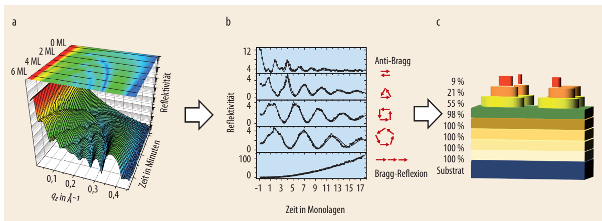
Abb. 4 Röntgenreflektivität während des Kristallwachstums von Diindenoperylen (DIP) auf Siliziumdioxid (a). Die Intensität bei festen q_z -Werten wie 1/2 q_{\text{Bragg}} (Anti-Bragg-Punkt) bzw. a q_{\text{Bragg}} ( a = 2/3, 3/4 und 4/5 ) oszilliert als Funktion der Zeit (b, die Zeit ist hier in eine Schichtdicke übersetzt). Die Periodizität lässt sich als Vektoraddition der komplexen Streuamplituden
